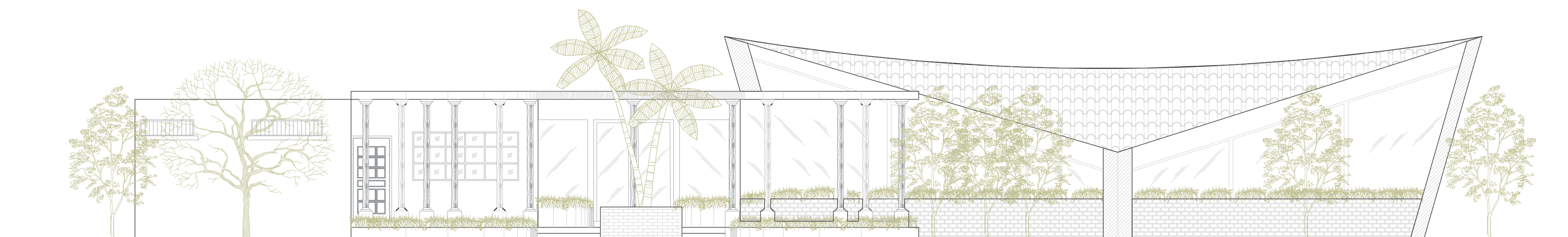
Section A-A
