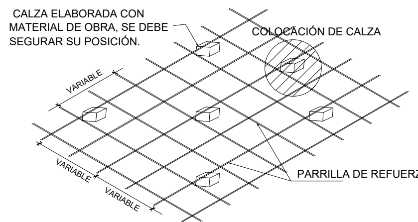
DETALLE TIPO DE COLOCACION DE CALZAS EN TRESBOLILLO PARA PARRILLA
