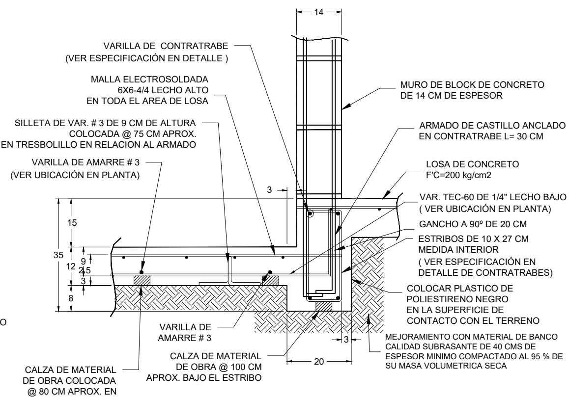
DETALLE 6-6' DE CONTRATRABE PERIMETRAL REDUCIDA
