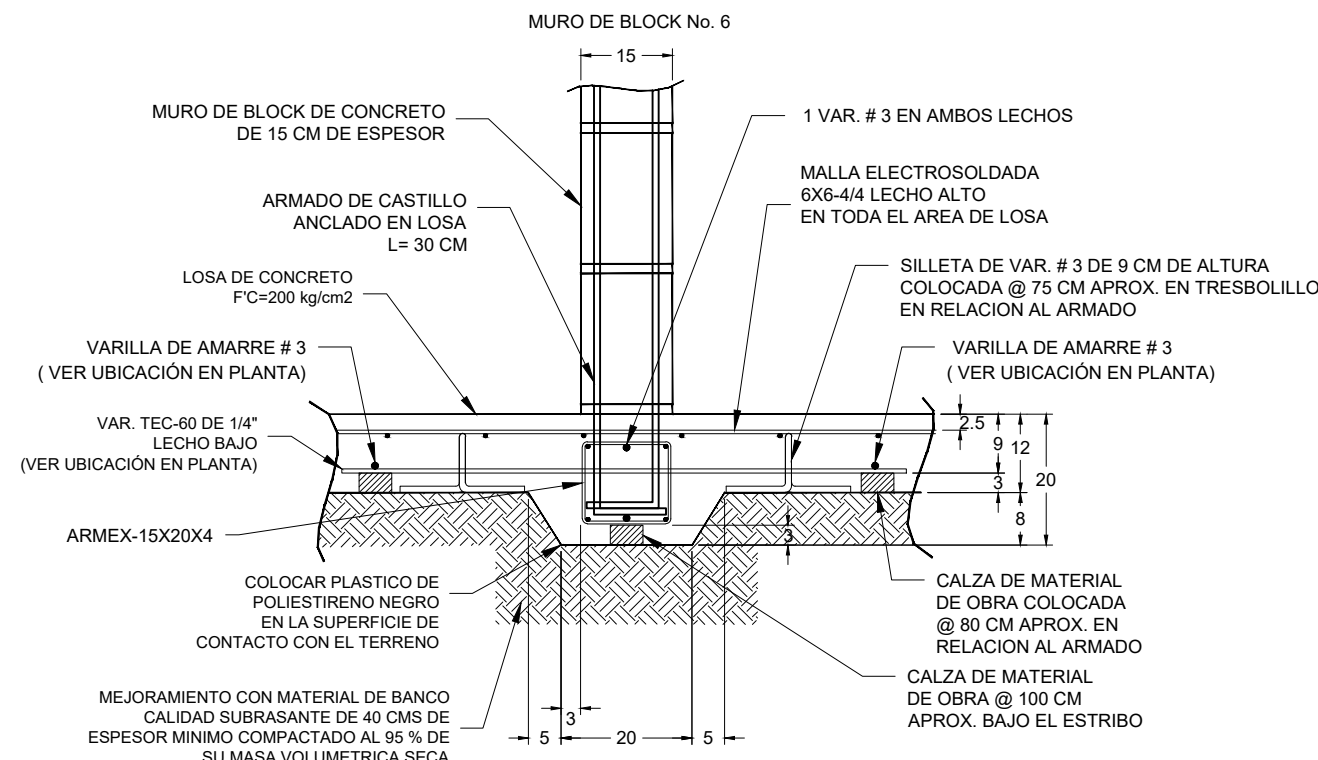
SOBRE ANCHO EN MUROS DIVISORIOS
