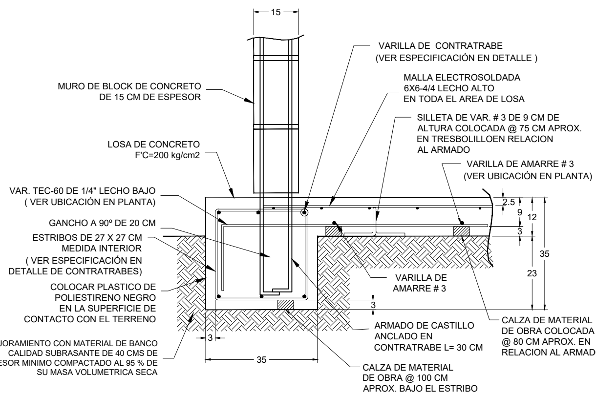
DETALLE 4-4' DE CONTRATRABE PERIMETRAL
