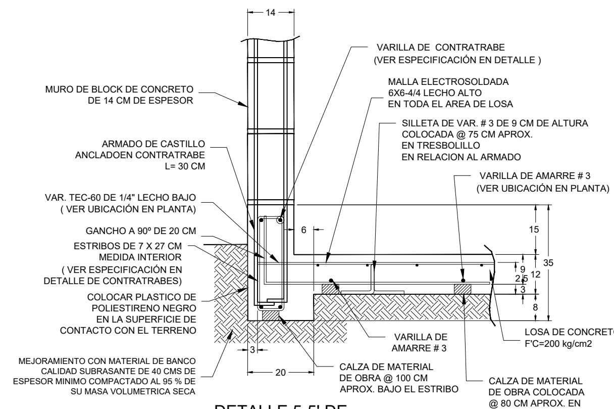
DETALLE 5-5' DE CONTRATRABE PERIMETRAL REDUCIDA
