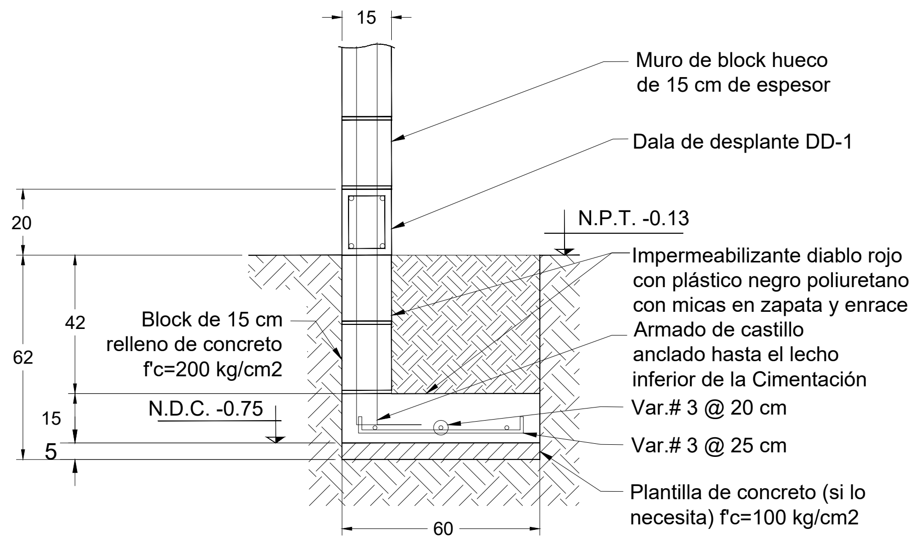
DETALLE 1-1' ZAPATA ZC-1
