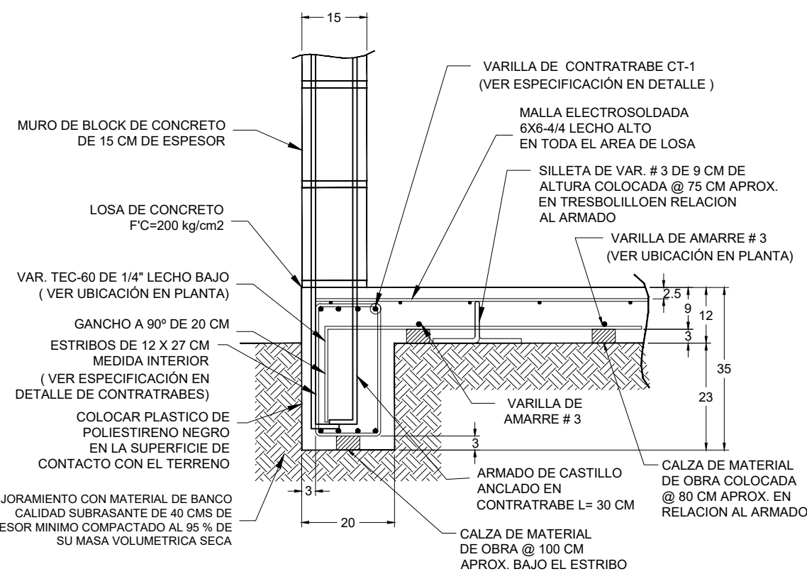
DETALLE 2-2' DE CONTRATRABE PERIMETRAL
