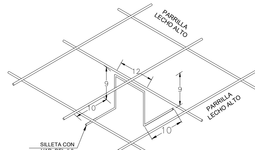
SILLETA PARA PARRILLA LECHO ALTO (SE CALZA EL HILO SUPERIOR)
