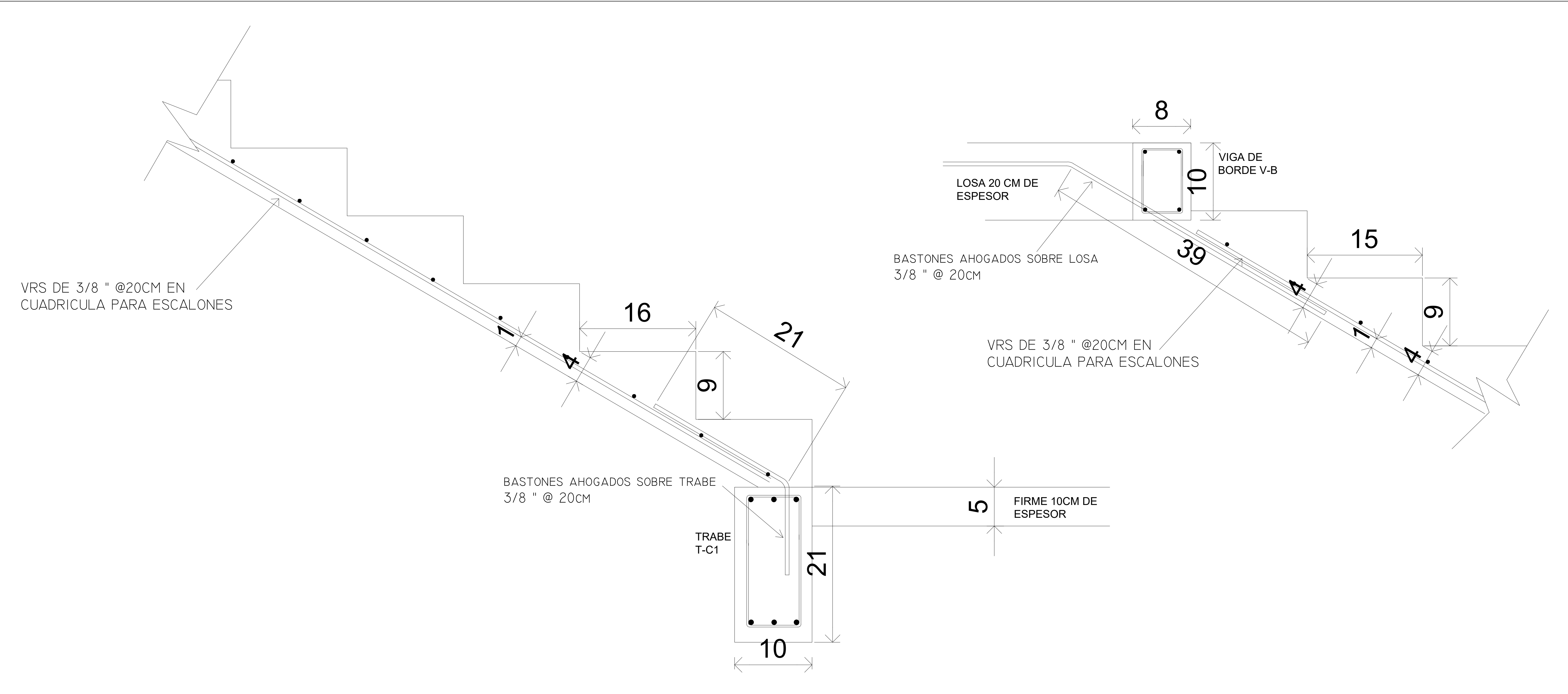
DETALLE ESTRUCTURAL DE ESCALERA DE CONCRETO STRUCTURAL DETAIL OF CONCRETE STAIR
