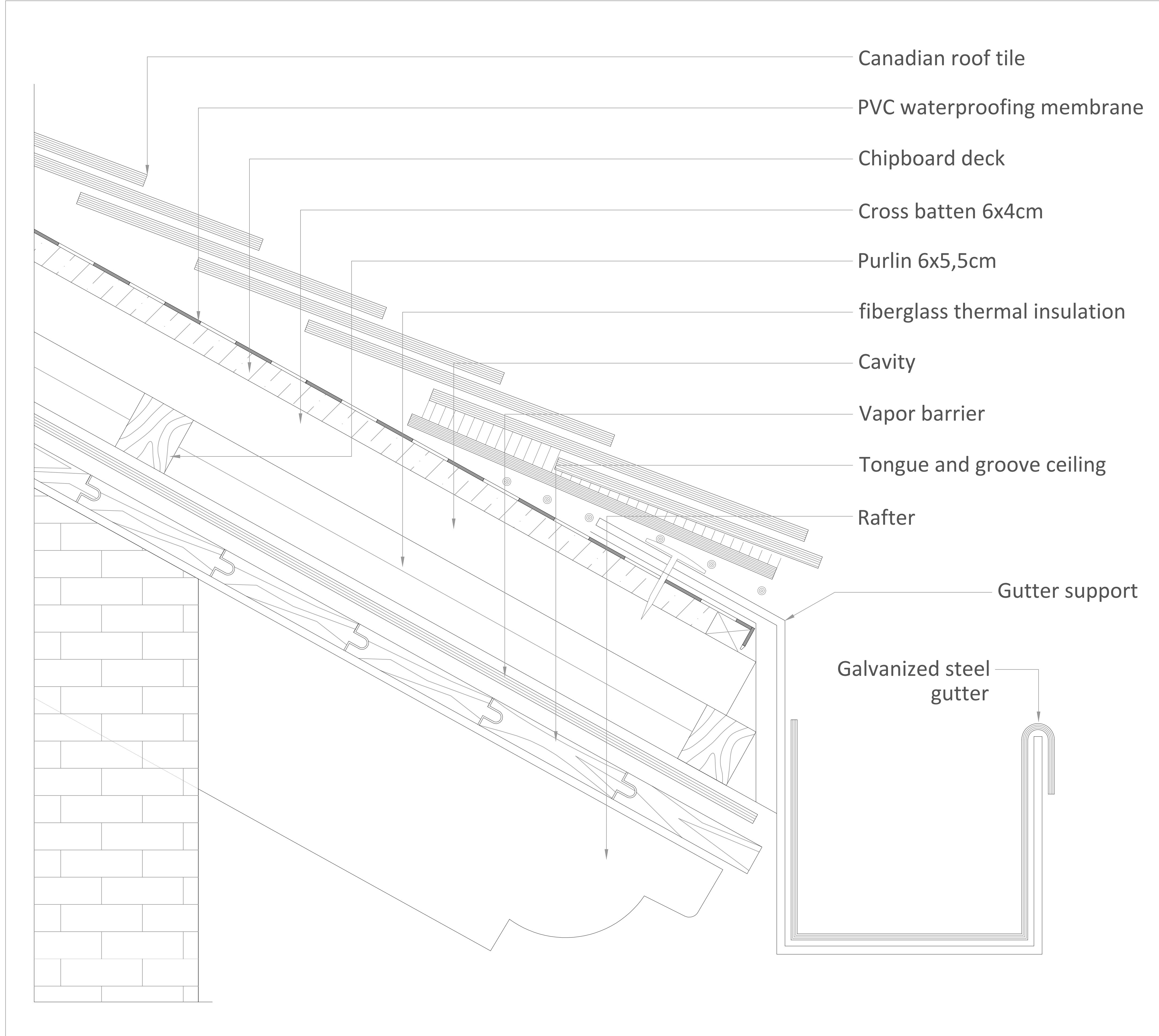
DETALLE CONSRUCTIVO DE CUBIERTA DE TEJA CONSTRUCTIVE DETAIL OF TILE ROOF
